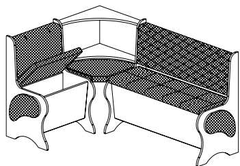
Кухонный уголок №1* 1532x1060x800
