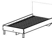
изд. 84.01 Каркас кровати 1925 × 942 × 336 матрац 1900 × 900
