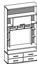
изд.7 1274 × 430 × 2250
