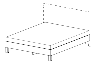
изд. 28.1M 2090 × 1654 × 960 матрас 2000 × 1600
