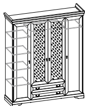
изд. 367 1914 × 580 × 2197
