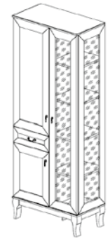
изд. 390пр Шкаф МФН 816 × 430 × 2016
