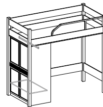
Кровать 2-х ярусная №4* 1986 × 984 × 1746 матрац 1900 × 900
