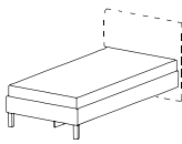
изд. 84.01 1925×942×336 матрас 1900×900
