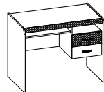
изд.3 1000 × 560 × 760
