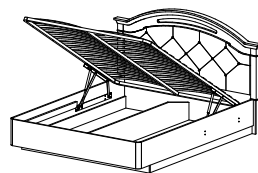
изд. 294м 1810 × 2075 × 1140
