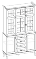
изд. 410 Буфет 1274 × 450 × 2060
