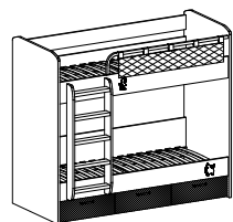
изд. №5 1954x886x1645 матрас 1900 x 800
