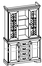
изд. 333 1264 × 450 × 2067
