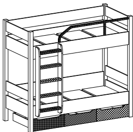
кровать 2-х ярусная №3 1944 × 884 × 1640 матраци 1860 × 800
