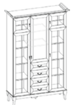
изд. 408 Шкаф МФН 1356 × 460 × 2060
